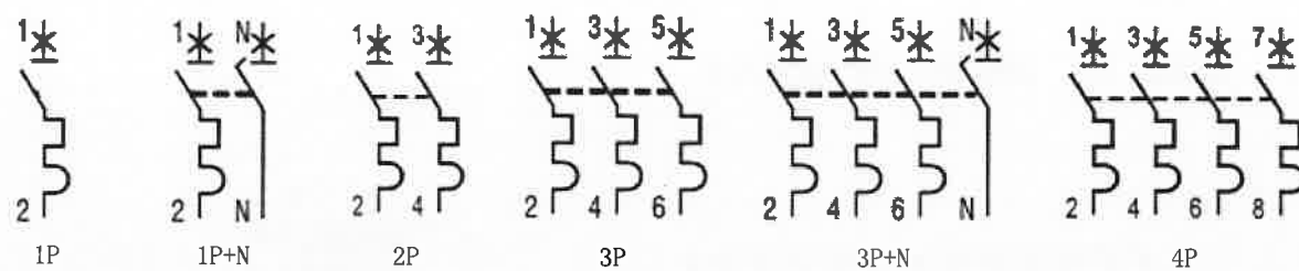
图1 线路图
